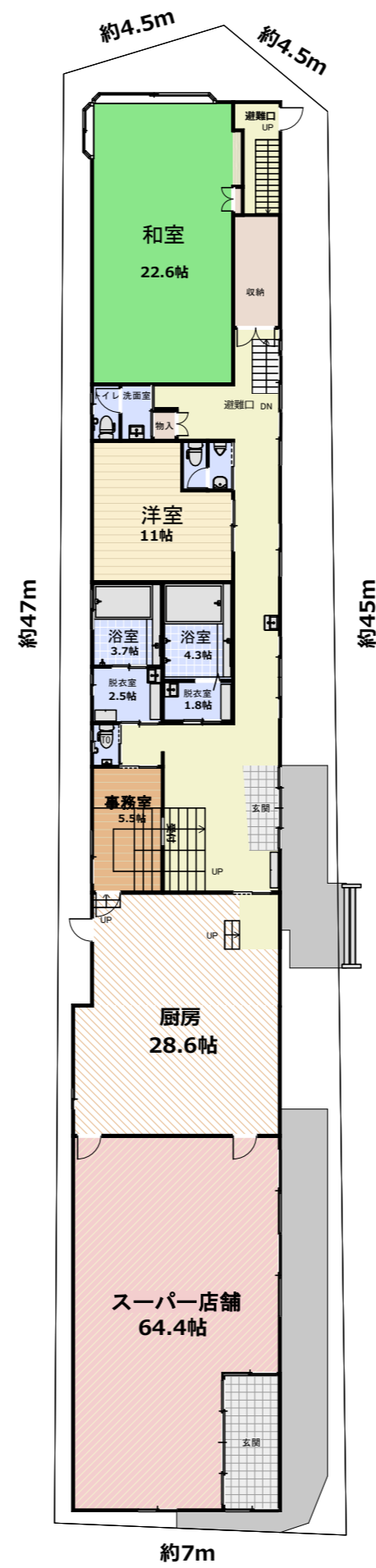
1階 縮尺 1/200
